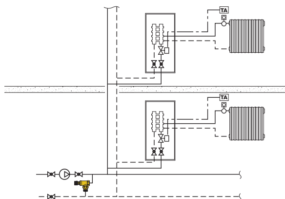
Impianto di piccole-medie dimensioni, by-pass in centrale
