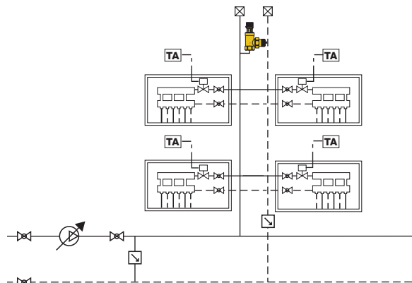
Impianto di medie-grandi dimensioni, by-pass in cima alle colonne
