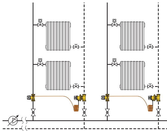
Controllo \Delta p su impianti a colonne
