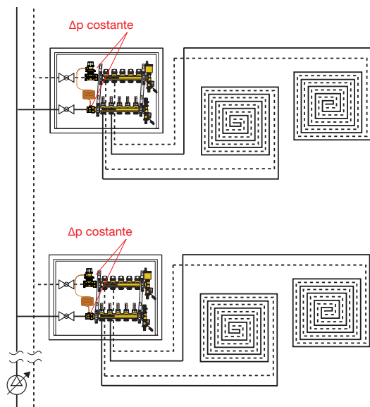
Controllo \Delta p su impianti a collettori
